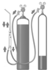
Топливный газ Кислород
