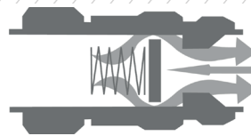
Обратный поток: опасная ситуация
